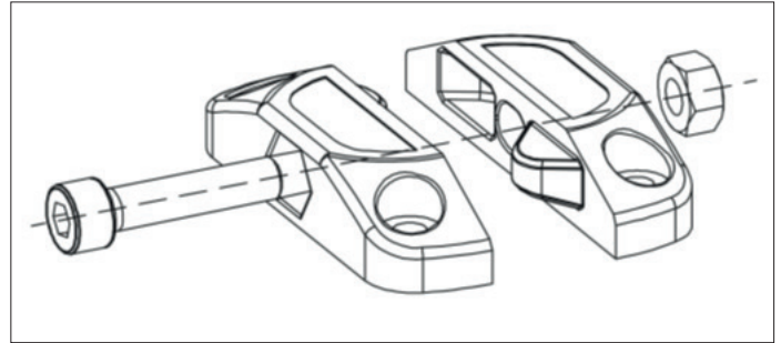
Şekil 17. Hücre birleştirme parçaları
