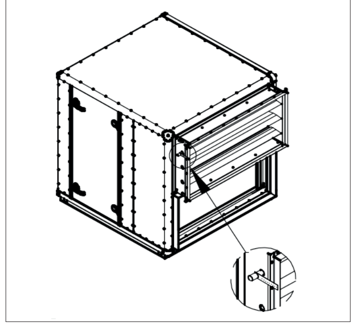
Şekil 56. Manuel çalıştırma
