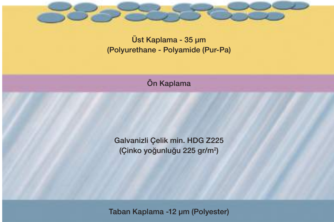
Panel kaplaması
