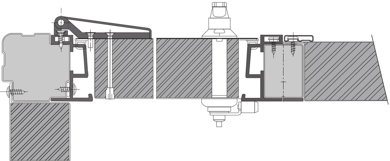
Kapı kesidi
